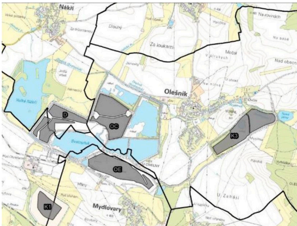
Obr. 2 – plánované plochy pro výstavbu solárního parku
